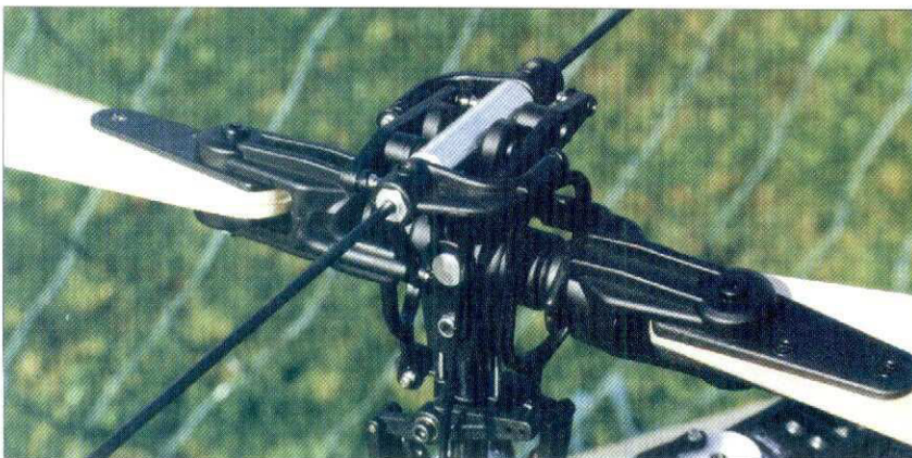
Raptor's rotorhuvud.
