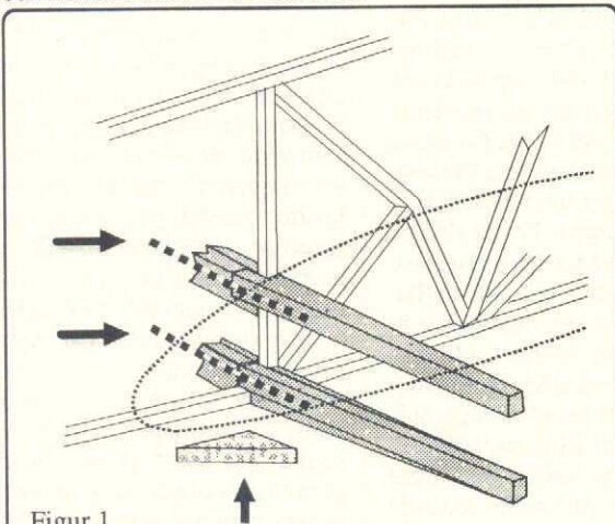
Figur 1 De punkterade linjer som pilarna pekar på visar vingbalkens svagaste del. Där bör man göra en förstärkning enligt vad som angivits i texten. Pilen på skissens undersida pekar på en ytterligare förstärkning. På flera platser vid vingmittbalkarnas infästning i kroppen kan man limma hörnskivor av till exempel 3 mm balsa. På den här platsen är det också lämpligt att utforma denna skiva så att den stöder V1, sprygels framkant.
