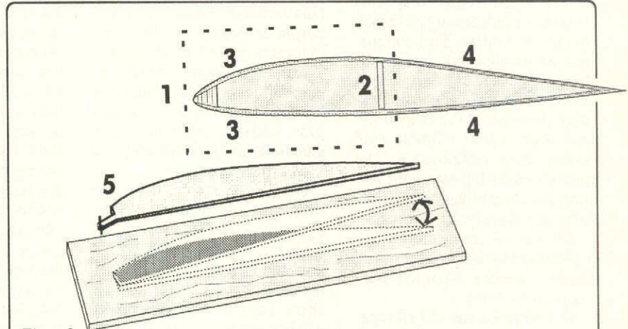
Figur 2 Området innanför den streckade ramen på profilsnittet utgör vingens "låda". Delarna i lådan är #1 framkant, #2 web, #3 beklädnad, (på Klemm är #1 och #2 mittbalkar). Vingskissen gäller för modellen Ogar som beskrivs i texten. Webbarna är de stående "listerna" mellan spryglarna. Bakkanten består av två smala balsaflak. Capstrips #4 med längsgående fiberriktning. Sprygel tillverkningen för denna vingtyp blir enkel. Sprygelmallen #5 har ett stift i främre delen. När man vrider mallen kan man skära ut spryglar i olika längder. Denna idé för sprygel tillverkning är gammal och det har påtalats tveksamheter huruvida det skulle bli rätt profil. Även jag har haft vissa tvivel, men vet nu, efter simulering i dator, att det ger perfekt resultat.
