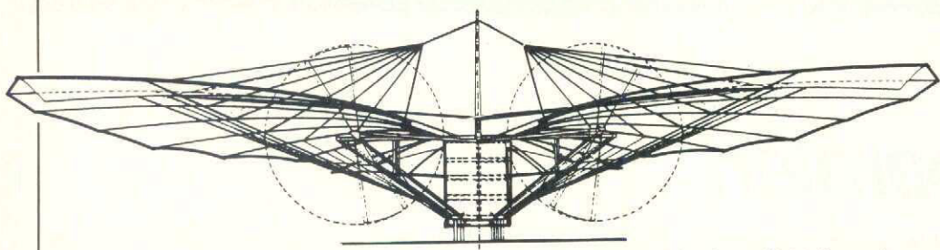
Drivenheten till de två propellrarna
